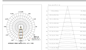
45°-3000K-CRI90
