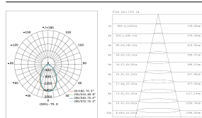
70°-3000K-CRI90
